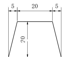
目地部詳細図 (S=1/1)
